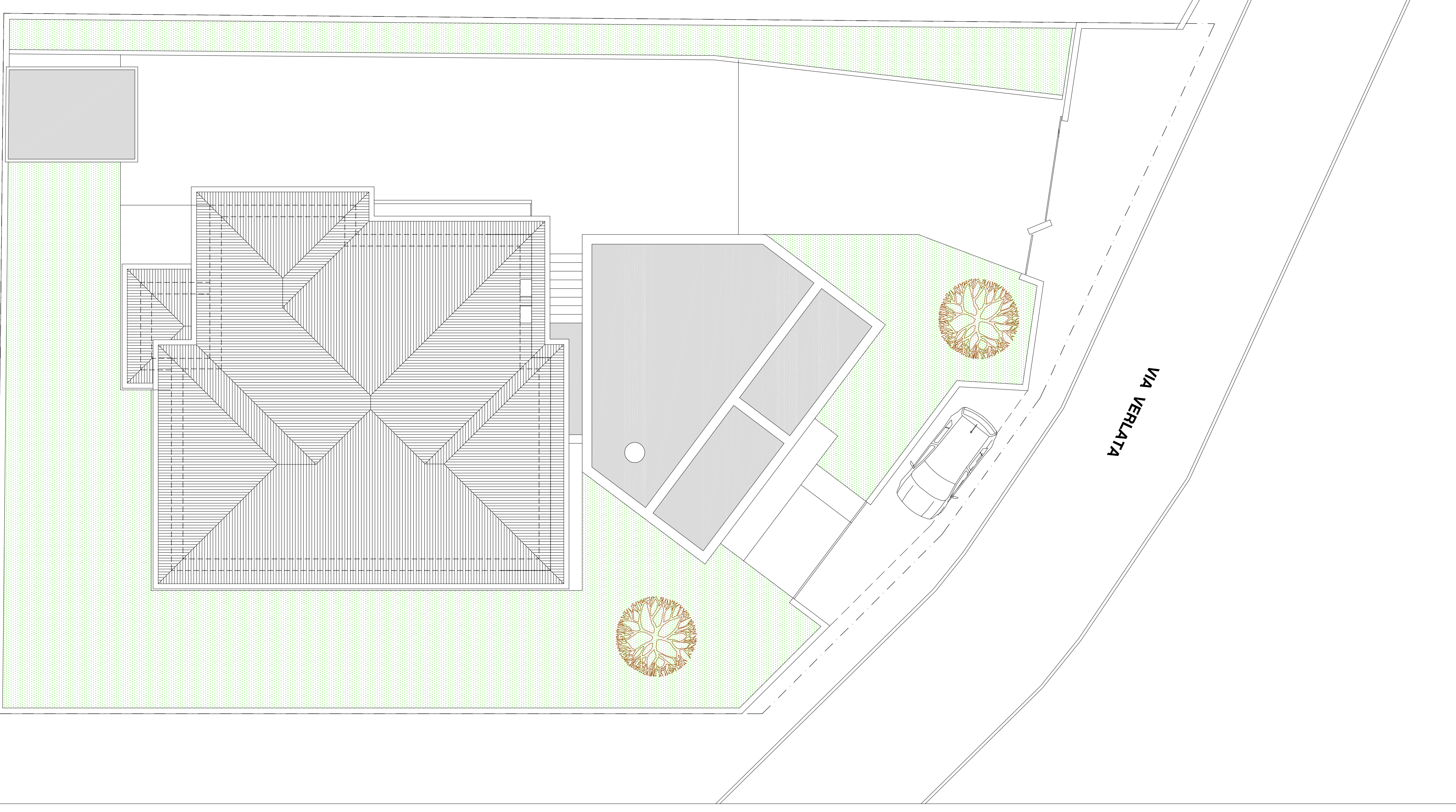
PIANTA COPERTURE
