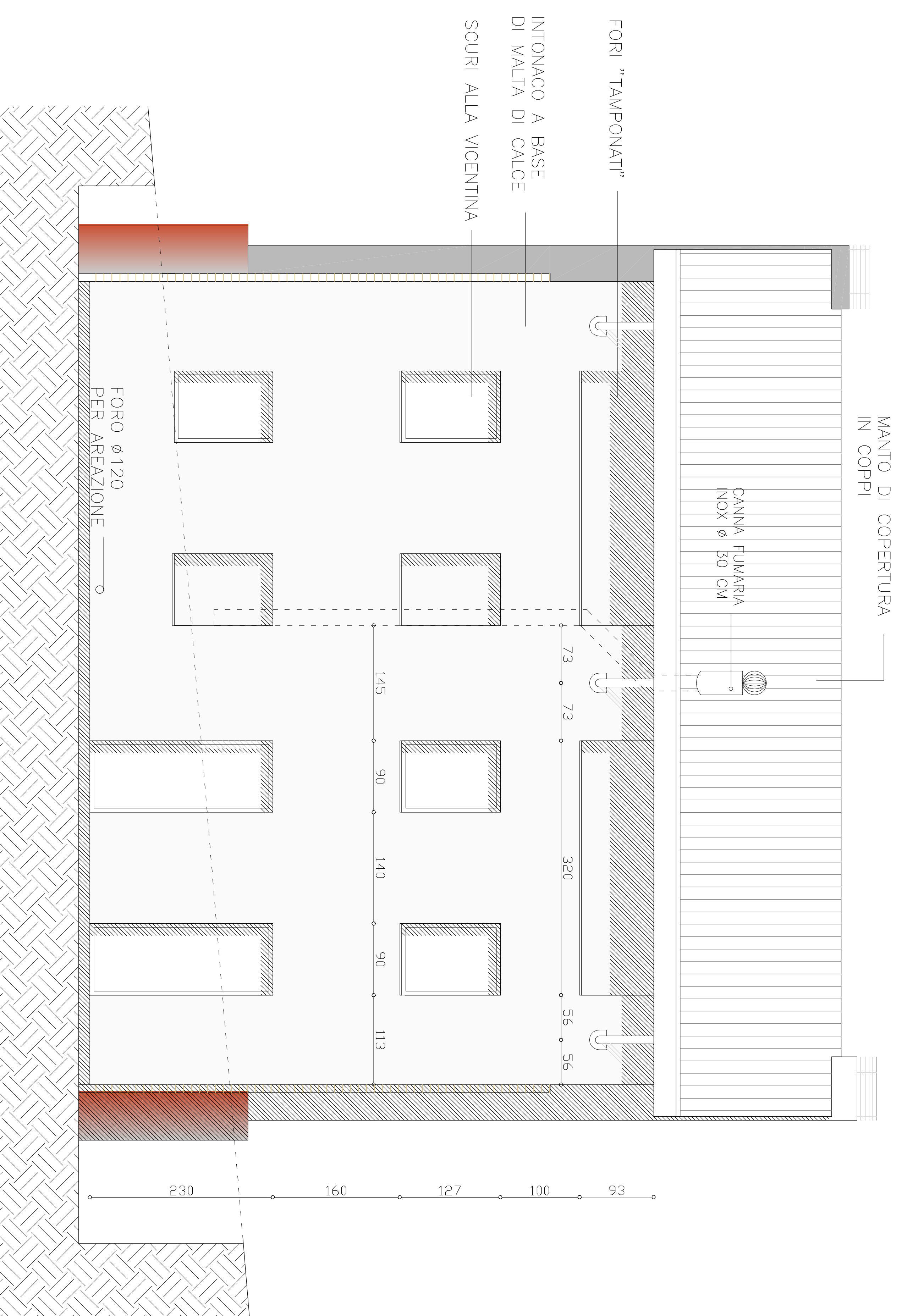
PROSPETTO NORD
