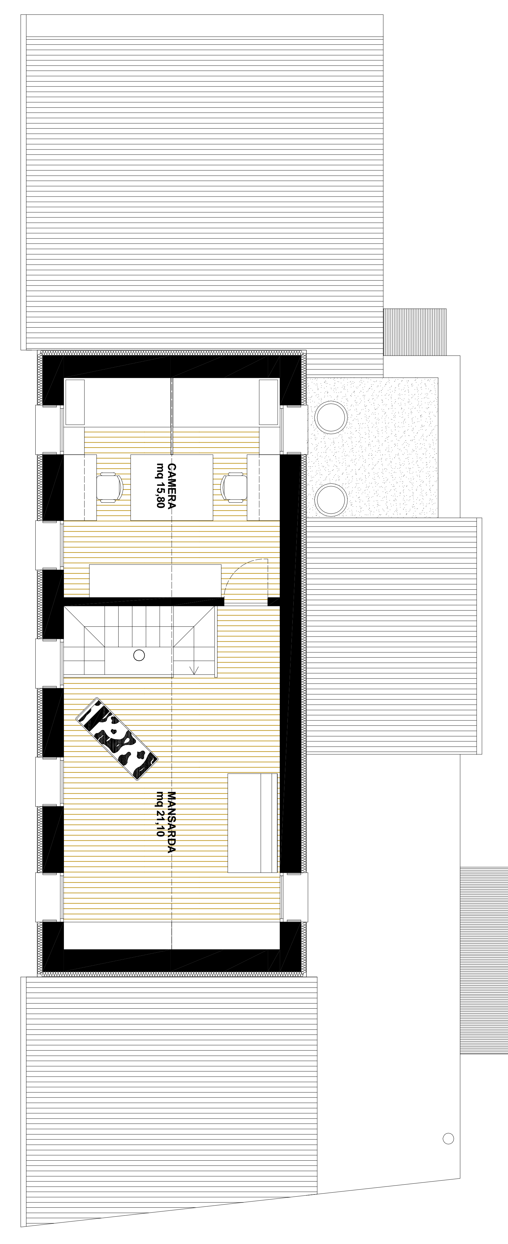
PIANTA PIANO SECONDO
