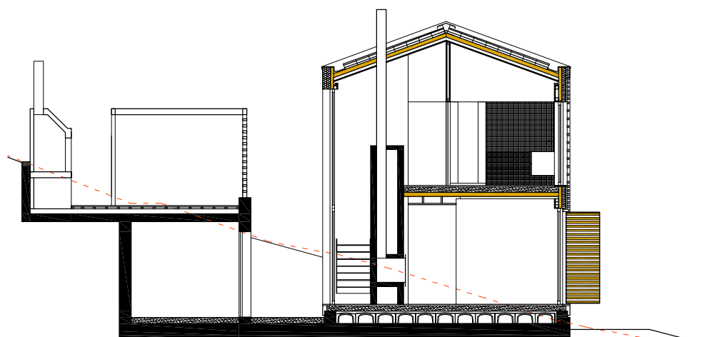
SEZIONE TRASVERSALE EE
