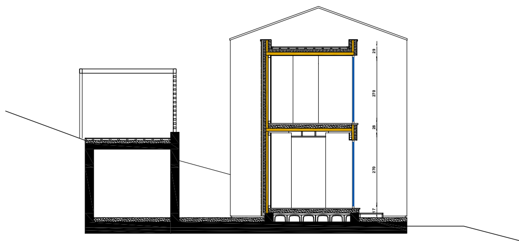
SEZIONE TRASVERSALE DD
