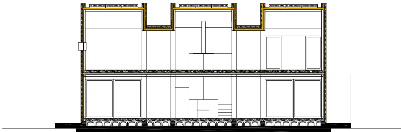
SEZIONE LONGITUDINALE AA
