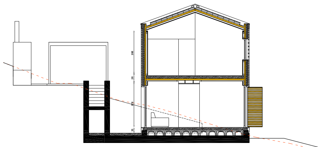
SEZIONE TRASVERSALE CC
